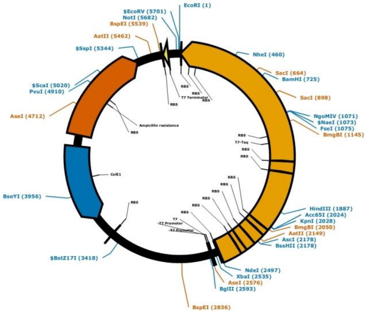
pET-Taq 5708 bp
